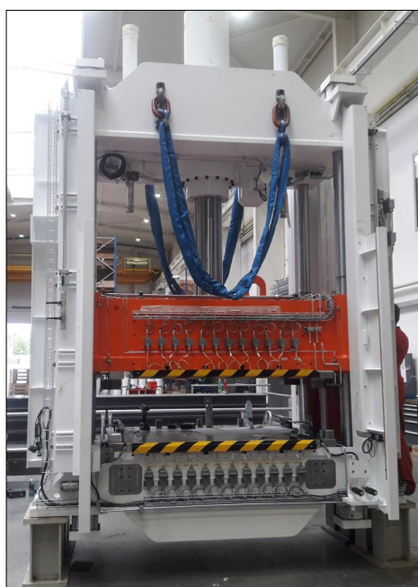
Celkový pohled na lis
