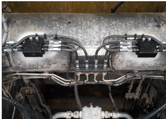
Sekundární progresivní rozdělovače SSV
