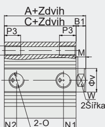
Typ se závitem
