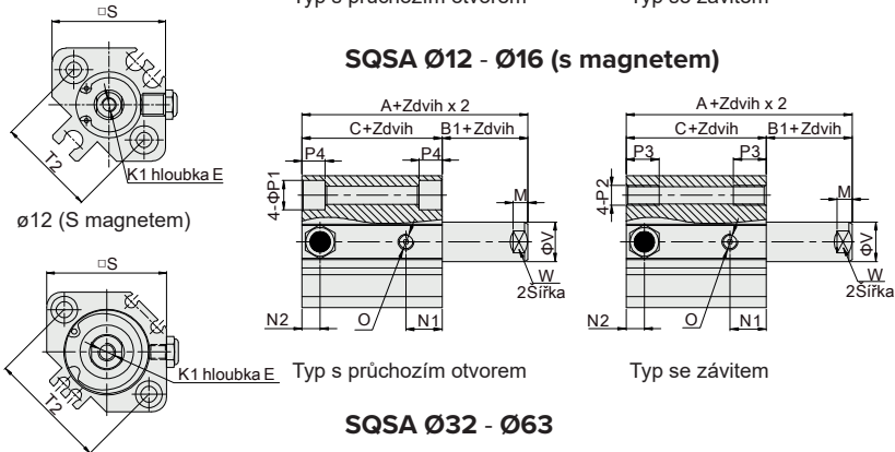
Typ s průchozím otvorem
