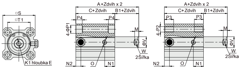
Typ s průchozím otvorem
