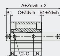
Typ s průchozím otvorem
