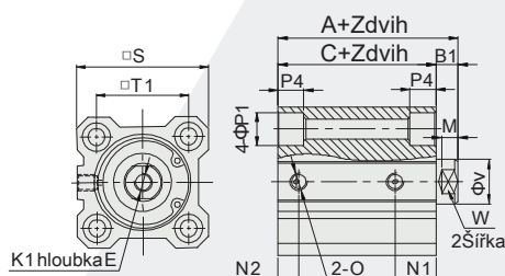
Typ s průchozím otvorem
