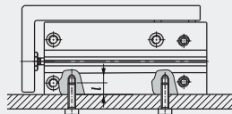
Svislé upevnění (závitové otvory)
