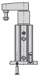
Upevnění dolní
