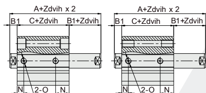
Typ s průchozím otvorem
