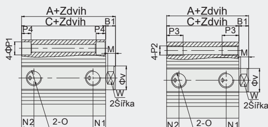
Typ s průchozím otvorem
