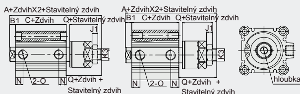
Typ s průchozím otvorem
