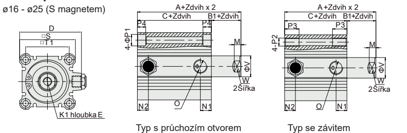
Typ s průchozím otvorem
