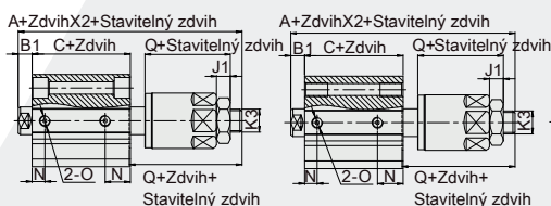
Typ s průchozím otvorem
