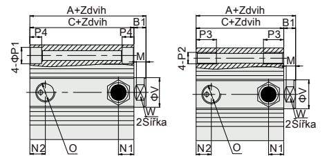
Typ s průchozím otvorem
