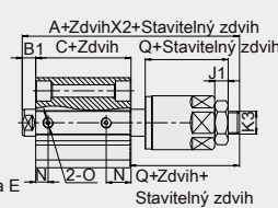
Typ s průchozím otvorem
