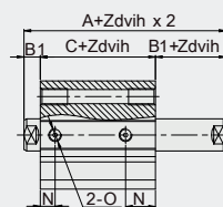
Typ se závitem
