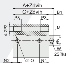
Typ se závitem
