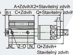
Typ se závitem
