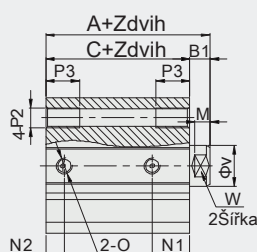
Typ se závitem
