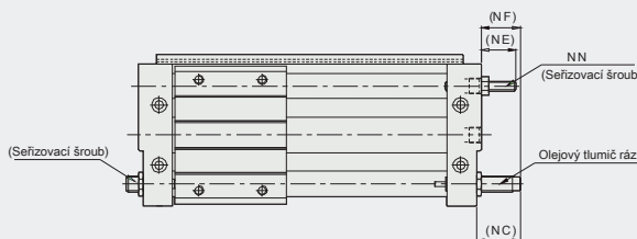
Se seřizovacím šroubem a olejovým tlumičem rázů
