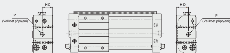
S olejovým tlumičem rázů
