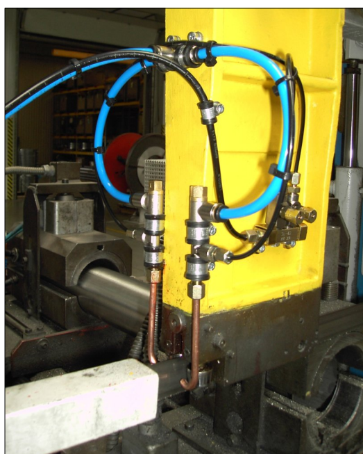
Celkový pohled na pilu
