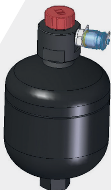
Membránový akumulátor S mini-měřícím připojením Případně 1/4" vnitřním závitem
