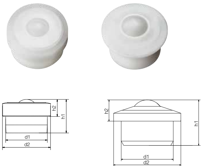
BB-505(B)-B180-POM BB-515(B)-B180-POM BB-522(B)-B180-POM
