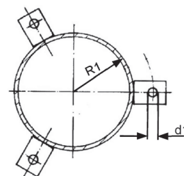
Obr. 7: Nohy pro DN 80 - 300
