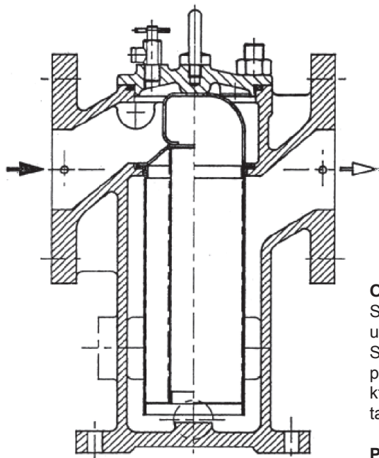
Obr. 1: Typ F118S (kryt se šrouby a maticemi)
