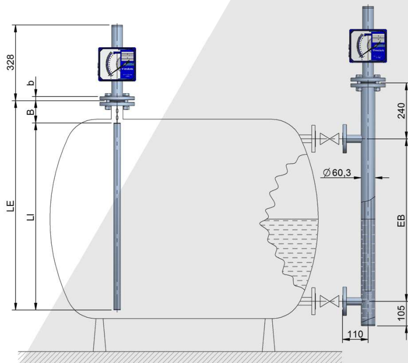
LP80 Montáž na horní část nádrže
