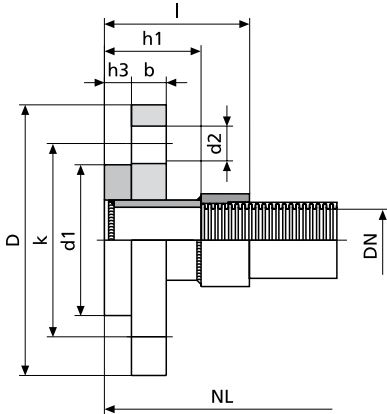
Loose flange PN 40 DIN 2656
