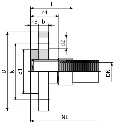
Loose flange PN 64 DIN 2636 (similar)
