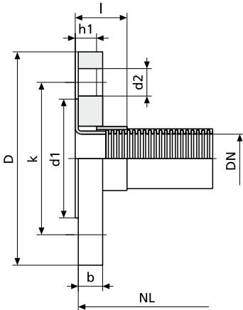
Loose flange PN 10/16 DIN 2642
