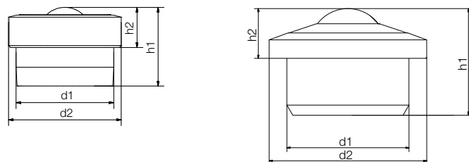
BB-505(B)-B180-POM
