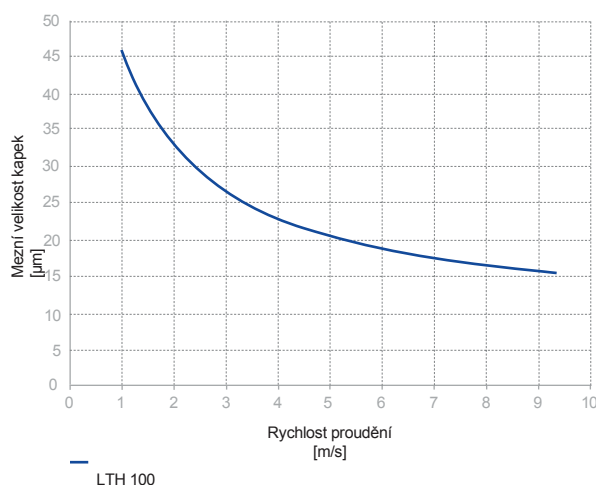
LTH 100 diagram mezních kapek
