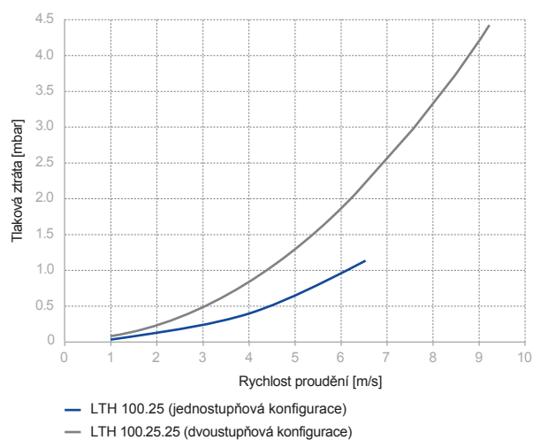
Diagram tlakových ztrát LTH 100
