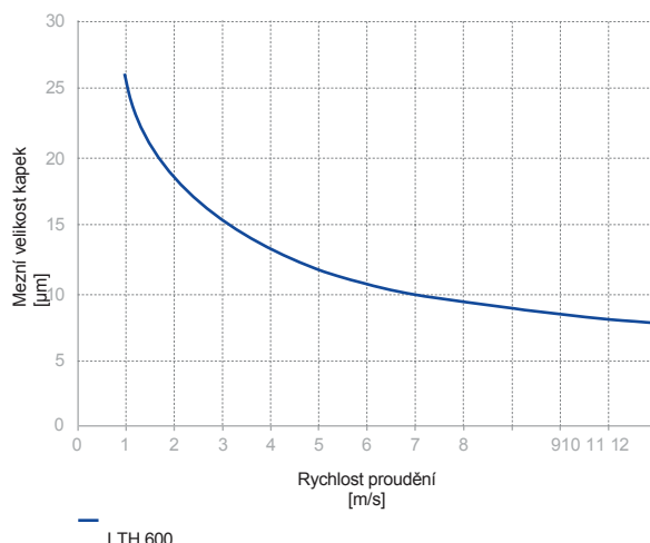
Hraniční diagram kapek LTH 600
