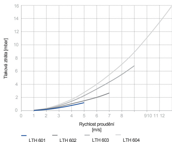
Diagram tlakových ztrát LTH 600
