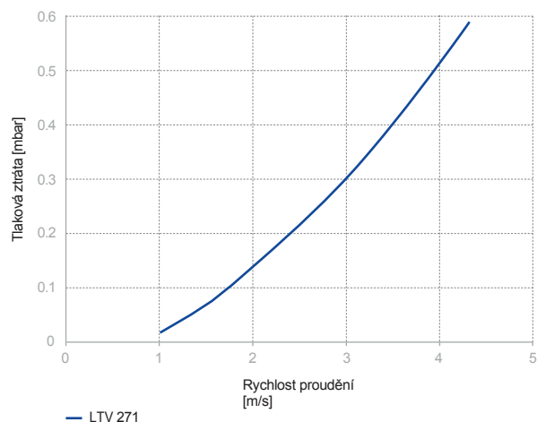
Diagram tlakových ztrát LTV 271
