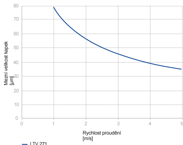
LTV 271 diagram mezních kapek
