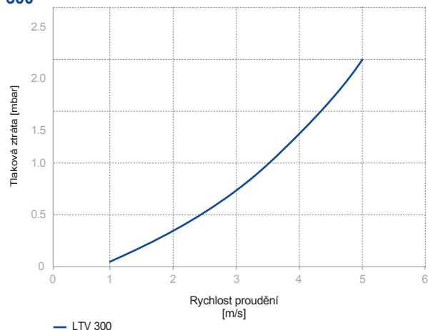
Diagram tlakových ztrát LTV 300
