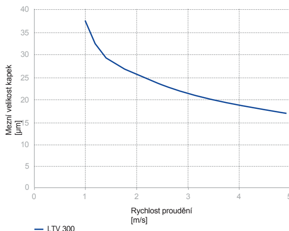
Hraniční diagram kapek LTV 300
