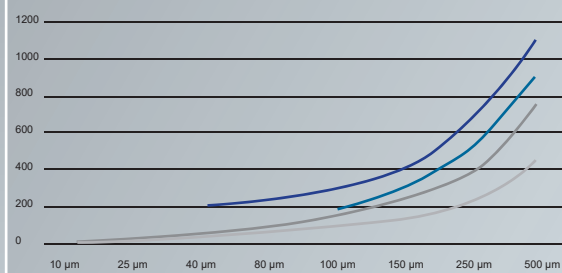
Závislost velikosti síta na míře znečištění TSS (mg/l)
