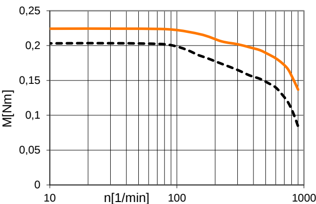
flange dimension 60 (NEMA24) MOT-AN-S-060-016-060-...
