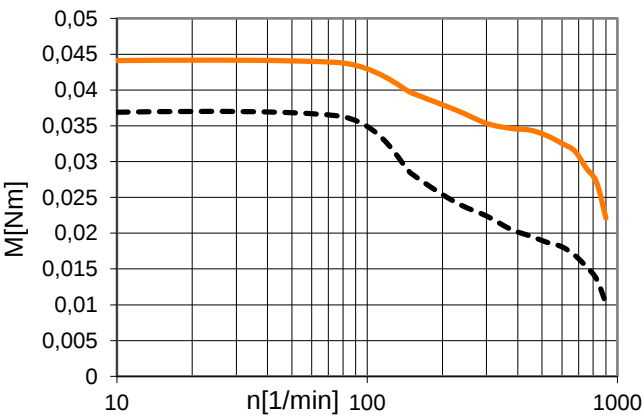
flange dimension 56 (NEMA23) MOT-AN-S-060-010-056-...
