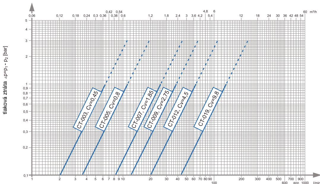
Průtokový diagram pro vodu při 20°C
