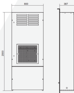
Rozměry
