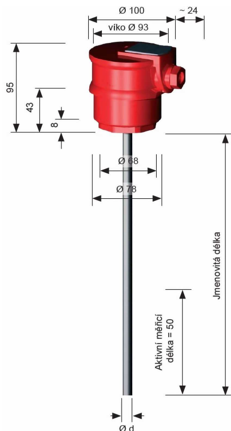
Teplotní snímač s pouzdem svorkovnice BC
