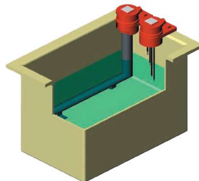
ORIENTAČNÍ TABULKA VODIVOSTNÍCH SOND JAKO OCHRANA PROTI CHODU NASUCHO PRO TRUBICOVÉ OHŘÍVAČE ROTKAPPE SE STANDARDNÍMI MINIMÁLNÍMI PONORY
