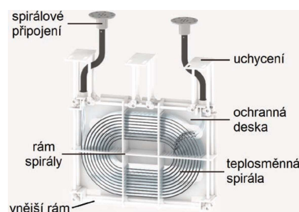
Spirálový polymerový výměník tepla SYNOTHERM®
