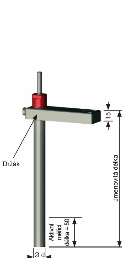
Teplotní snímač v provedení PG
