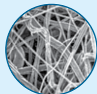
Vnitřní vrstvy polypropylenového materiálu pro finální filtraci
