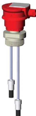
Vodivostní sonda NS se závitovou spojkou
