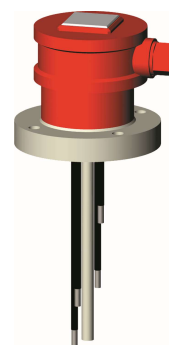
Vodivostní sonda NS se přírubou
